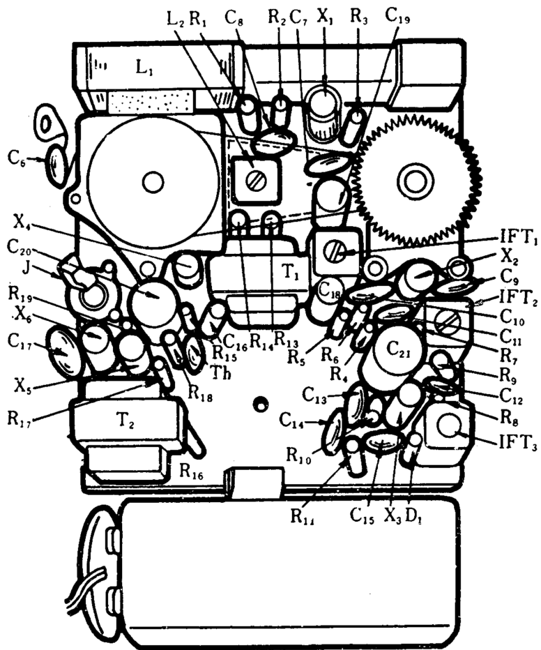
POSIZIONE DEI COMPONENTI (Telaio visto sul retro)
